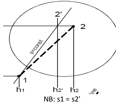
Fig. 16. Isentropic compressor.
