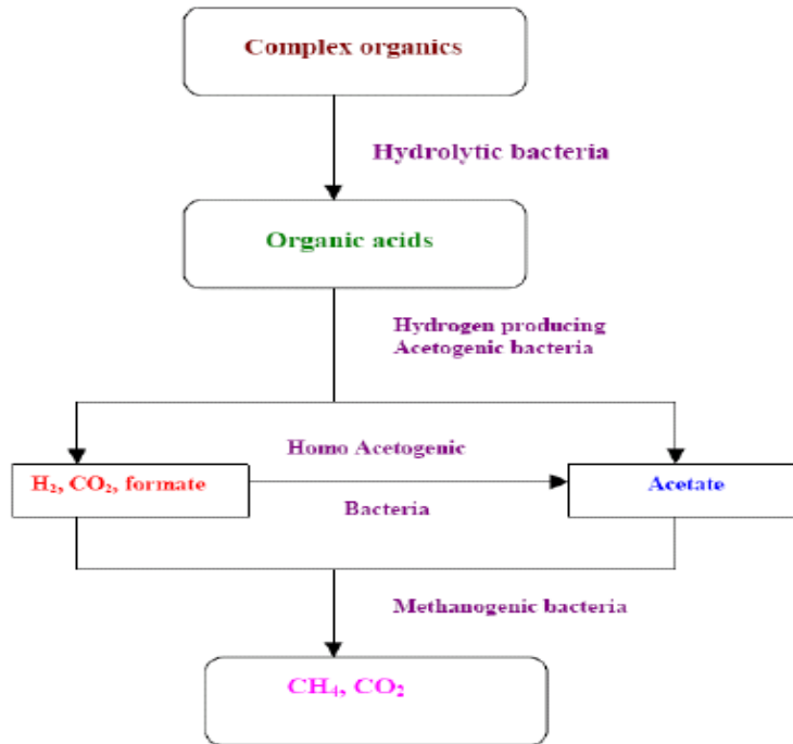
Fig. 3. Biogas production processes (Abdeen, 2012).
