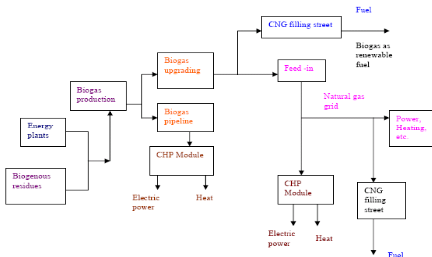
Fig. 4. Overview of biogas utilisation pathways (Omer, 2008).
